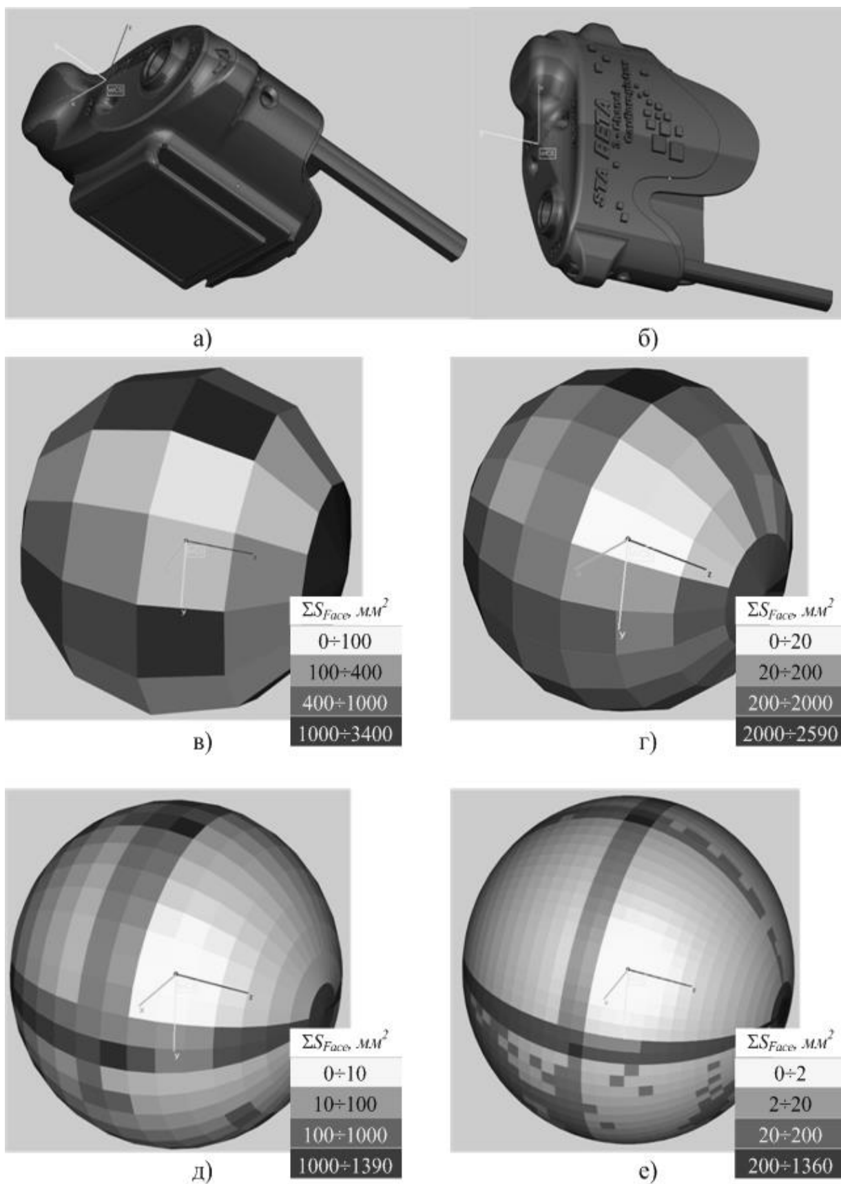
Рис. 4. Колірна візуалізація моделі кришки за коефіцієнтами одиничних векторів нормалей граней N_z (a) і N_y (б), відображенням на сферу сумарної площі граней при наступних інтервалах кутів нахилу вектора нормалі в сферичній системі координат: 30^\circ (в), 20^\circ (г), 10^\circ (д), 5^\circ (е)
