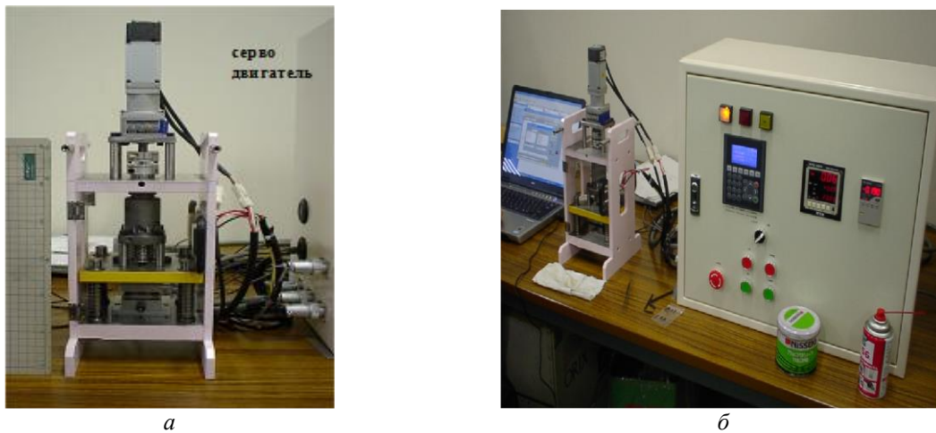
Рис. 6. Микронпресс (а) и микро-штамповка (б) (Nagoya Institute of Technology)
