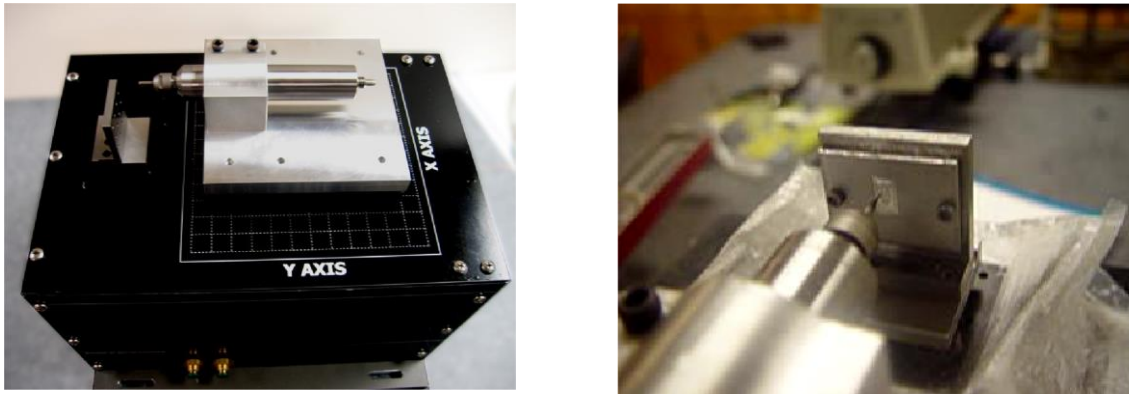
Рис. 3. Машини микро/мезо-размеров: рабочая зона 25×25×25 мм, подача 700 мм/с, скорость вращения инструмента 120К мин -1
