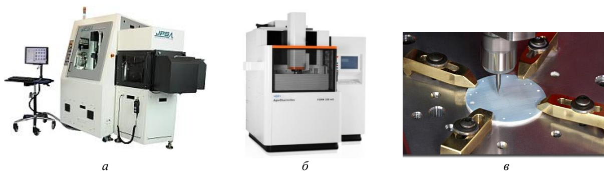
Рис. 2. Промышленные микро-машины: а – лазерная система; б – микро-EDM машина [3]; в – стенд для микро-сверления [8]
