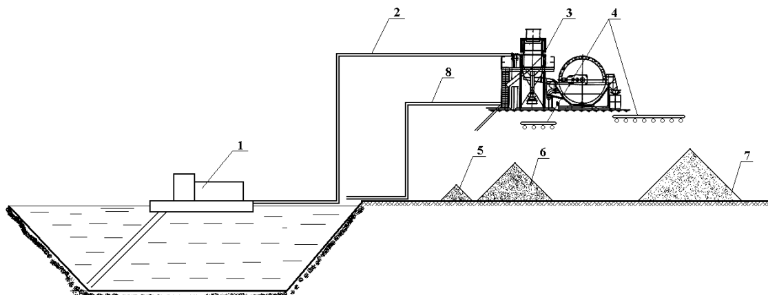
Рис. 1. Схема КВП «земснаряд–пульпопровід–класифікаційна установка»: 1 – землесосний снаряд; 2 – пульпопровід; 3 – класифікаційна установка; 4 – відвальні конвеєри; 5,6 – склади крупного і мілкового ґравію; 7 – склад товарного піску; 8 – патрубок відводу шламів
