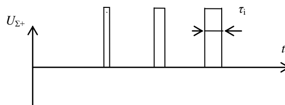
Рис. 5. Виділення позитивних імпульсів з виходу підсумовуючого пристрою
