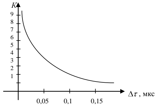
Рис. 7. Залежність коефіцієнта складності аналізатора тривалості імпульсів від точності їх вимірювання
