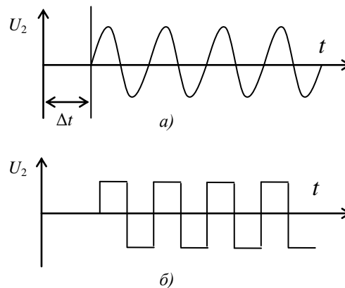
Рис. 3. Сигнал, прийнятий другим пунктом на вході (а) та на виході ПО (б)
