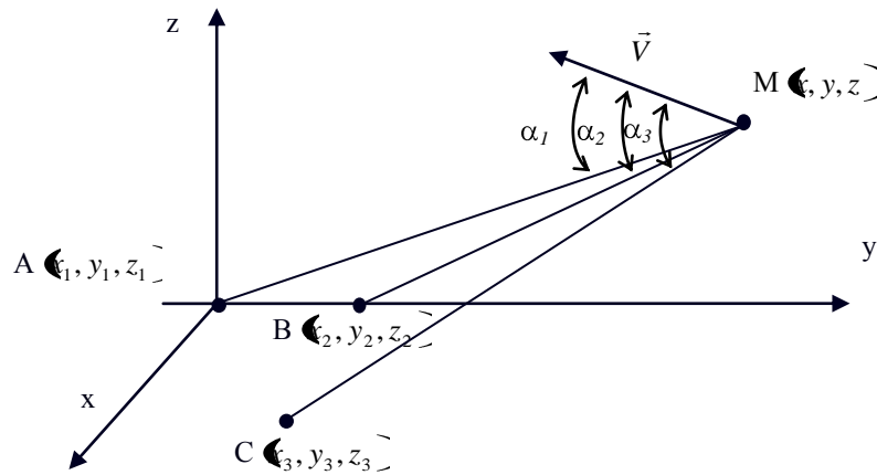
Рис. 1. Положення ДРВ відносно пунктів прийому РТС
