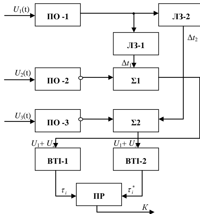
Рис. 6. Структурна схема вимірювача відношення різниці доплерівських частот
