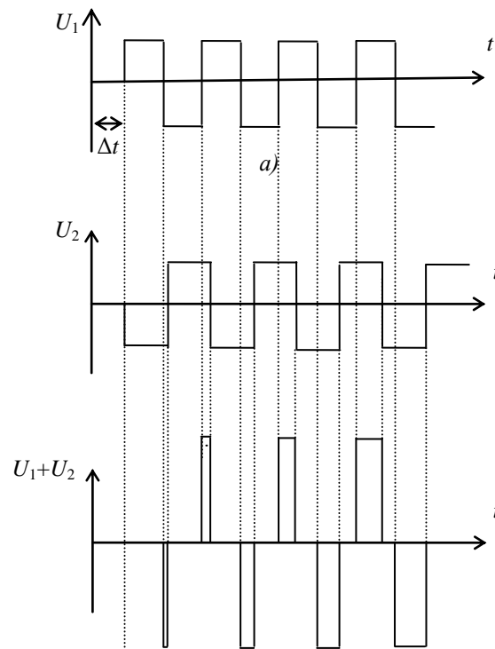
Рис. 4. Сигнали на вході (а) та на виході пристрою підсумовування
