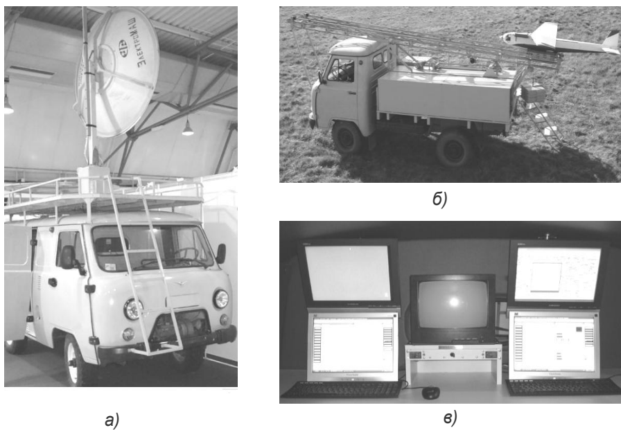
Рис. 3. БпАК “Грант”: а – машина управління; б – машина пуску; в – у середині машини управління
