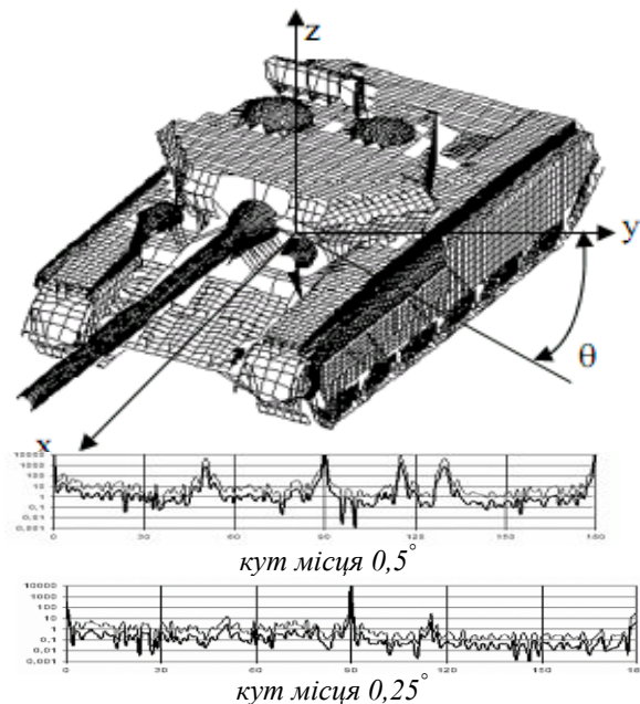
Рис. 7. Фасеточна модель танка Т-90 і його ЕПР на частоті 37,5 ГГц при куті місця 0,5^\circ і 0,25^\circ
