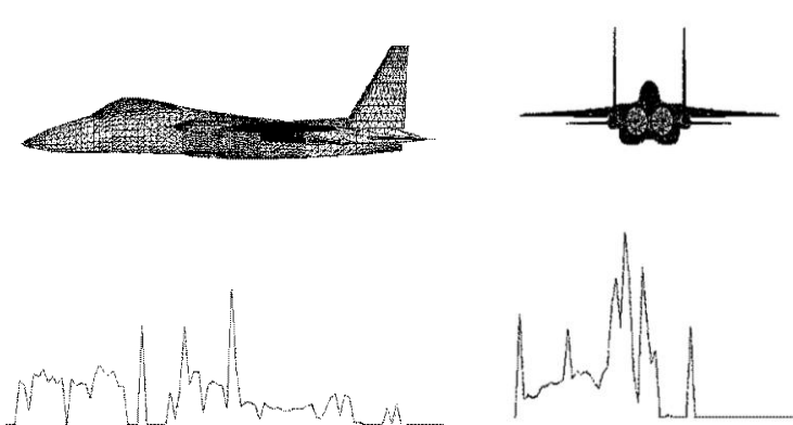
Рис. 4. “Фасеточна” модель літака Су-27 і діаграма ЕПР залежно від кута спостереження в горизонтальній площині
