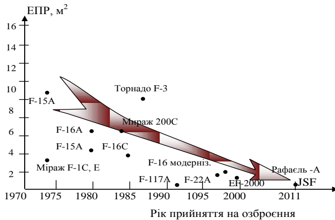
Рис. 1. Тенденції зміни радіолокаційної помітності надзвукових літаків
