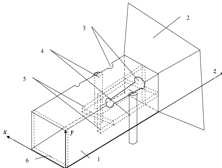
Рис. 8. Конструкція рупорної антени колової поляризації зі зменшеною ЕПР: 1 – хвилевід; 2 – розкрив рупора; 3 – гантелеподібні щілини; 4 – коаксіальне навантаження; 5 – діелектричні пластини для обертової поляризації; 6 – поглинаюча пластина
