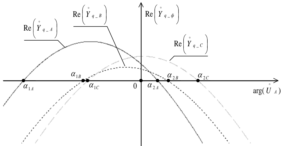
Рис. 2. Графіки функцій \operatorname{Re}(\dot{Y}_{q-\phi})\left(\arg(\dot{U}_A)\right) для фаз A, B, C в околі \arg(\dot{U}_A) = 0
