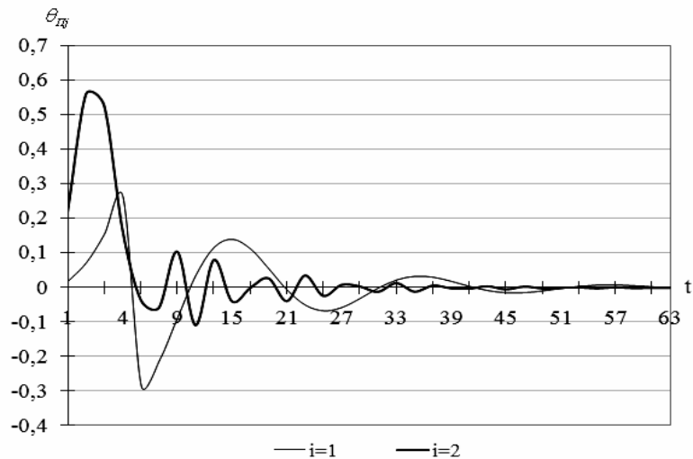
Рис. 2. Графік поперечно-кутових коливань платформи напівпричепа із вантажем 8470 кг при виконанні маневру "переставка" сідельним автопоїздом на швидкості 45 км/год.:
