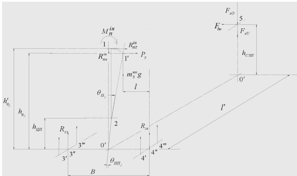
Рис. 3. Розрахункова схема сил, що діють на напівпричепу сідельного автопоїзда, з врахуванням поперечно-кутових коливань платформи напівпричепи і її нахилу на максимально можливий кут: R_{к\tau}^{3f} , R_{кн}^{3f} – тангенційна і нормальна складова головного вектора сили інерції; M_n^{3f} – головний момент сили інерції; P_y – сила інерції; F_{hw} , F_{so} , F_{su} – горизонтальна та вертикальна сили, що виникають у сідельно-зчипному пристрої; \theta_{пj} , \theta_{нпj} – кути крена підресорних та невідресорних мас
