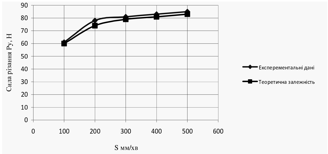
Рис. 2. Вплив повздовжньої подачі на силу різання, при V_0 = 20 м/хв., V_{кр} = 35 м/с, t = 0,2 мм, S = 300 мм/хв.
