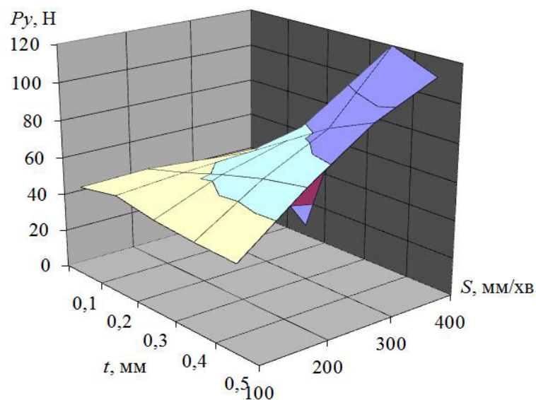
Рис. 3. Поверхня відгуку залежності радіальної сили різання P_y від повздовжньої подачі деталі та глибини різання кругом 1-600x500x305 14A25-Н С1-СМ2 7К1А 35 м/с з кількістю канавок 12 V_0 = 30 м/хв.
