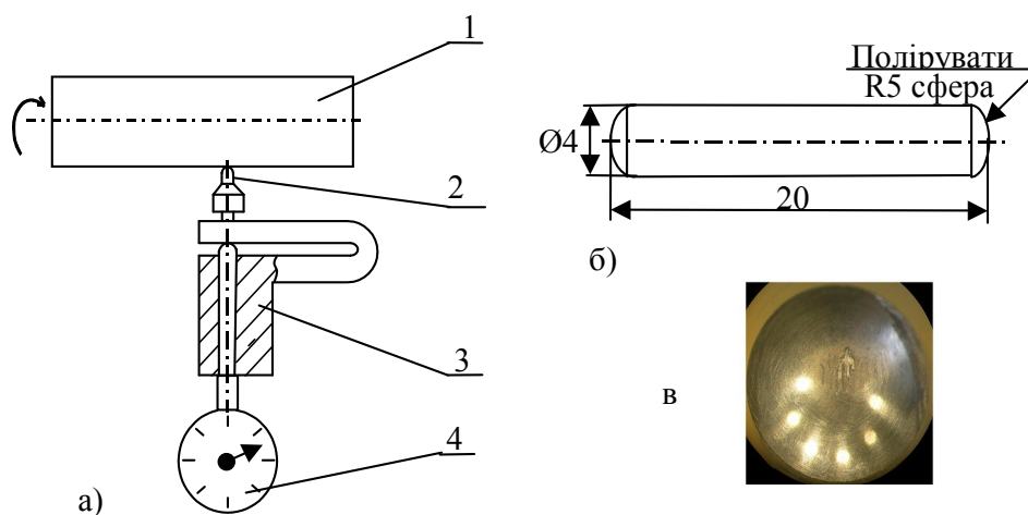
Рис. 1. Пристрій для попереднього дослідження екрануючих властивостей технологічних змащень: а) схема пристрою; б) деформуючий інструмент; в) торець стержня з налипом оброблюваного матеріалу
