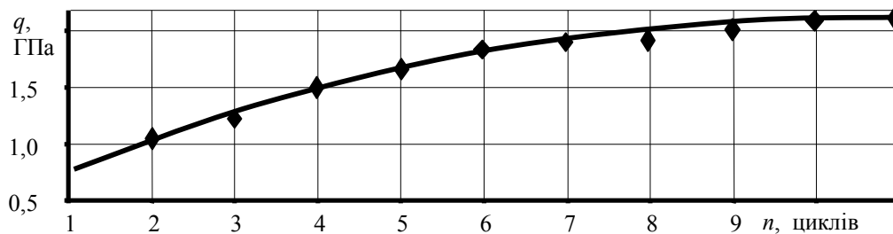
Рис. 4. Залежність контактної сили від кількості циклів деформування
