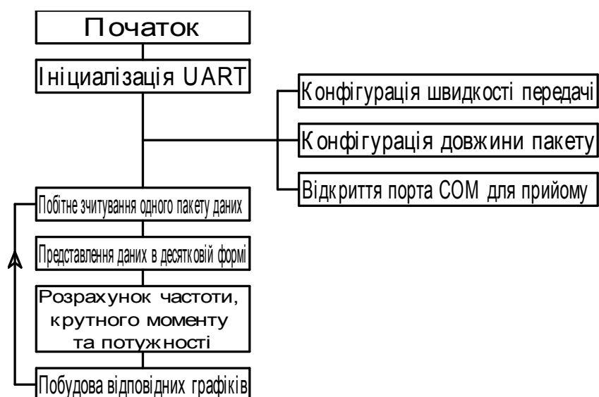
Рис. 9. Загальний алгоритм роботи програми «DTW»
