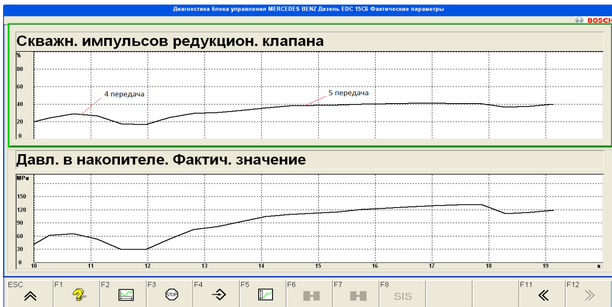
Рис. 2. Графіки зміни скважності сигналу регулятора та тиску палива в акумуляторі справно ПНВТ
