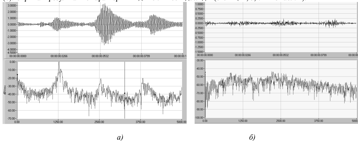
Рис. 2. Сигнал, записаний з п'єзоакселерометра, та спектрограма потужності сигналу без використання динамічного гасителя вібрацій (а) та з його використанням (б)
