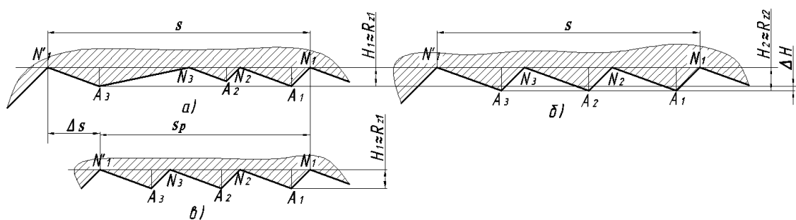
Рис. 7. Схеми розміщення різців: за запропованою методикою з подачею s та висотою мікронерівностей H_1 (а); традиційна з рівномірним розміщенням різців при забезпеченні подачі s та висоті мікронерівностей H_2 (б); традиційна з рівномірним розміщенням різців s_3 забезпеченням висоти мікронерівностей H_1 та зменшеною подачею s_p < s
