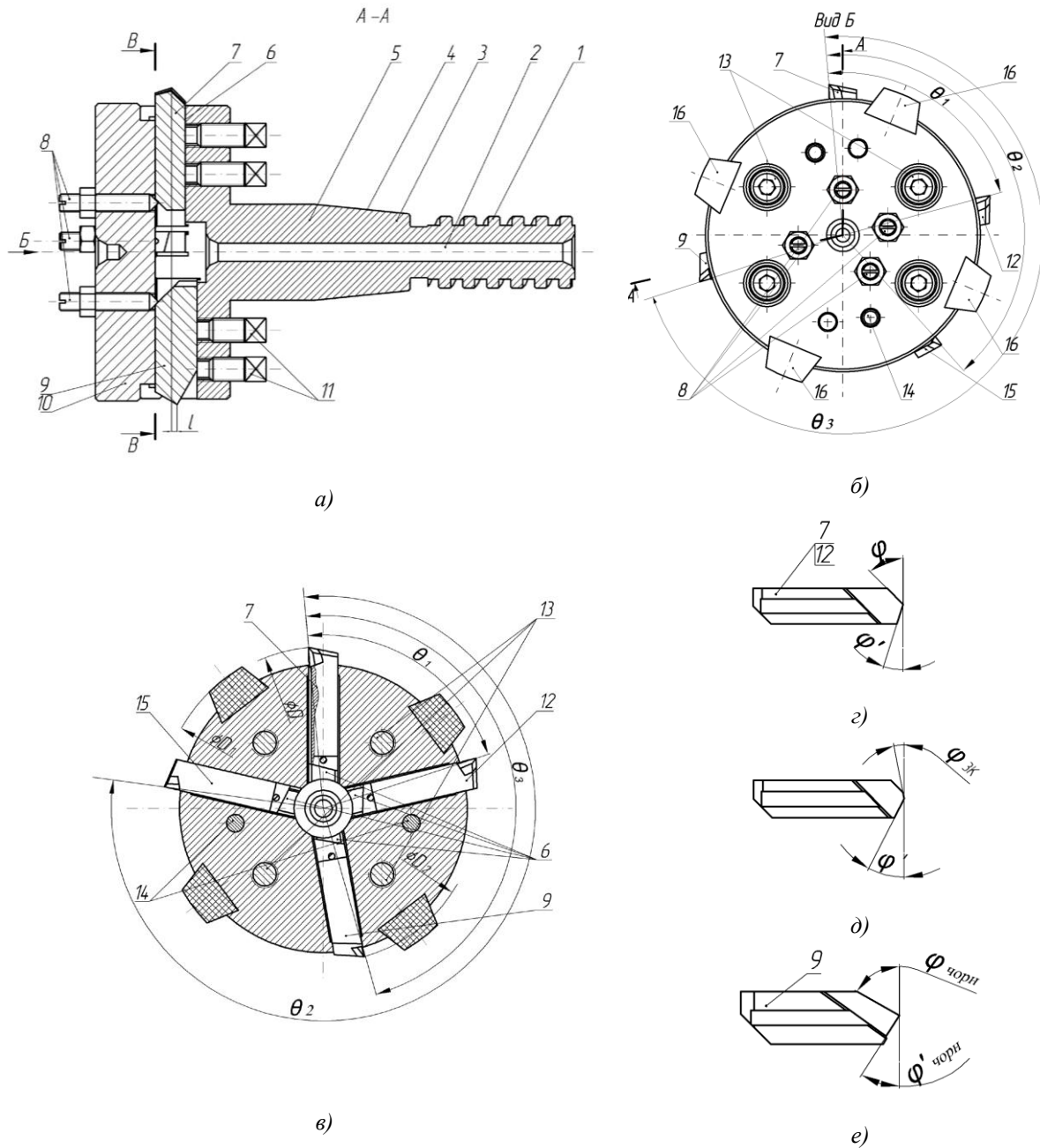
Рис. 4. Конструкція розточувальної головки для комбінованого розточування глибоких отворів за I варіантом конструкторського виконання: а – головний вигляд; б – вигляд по стрілі Б; в – переріз В-В; г, д, е – проєкції в плані відповідно першого та другого (г), третього (д) чистових і чорнового (е) різців
