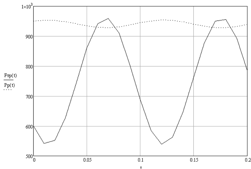
Рис. 6. Залежності сили тертя в контактї та дійсної сили тяги від часу
