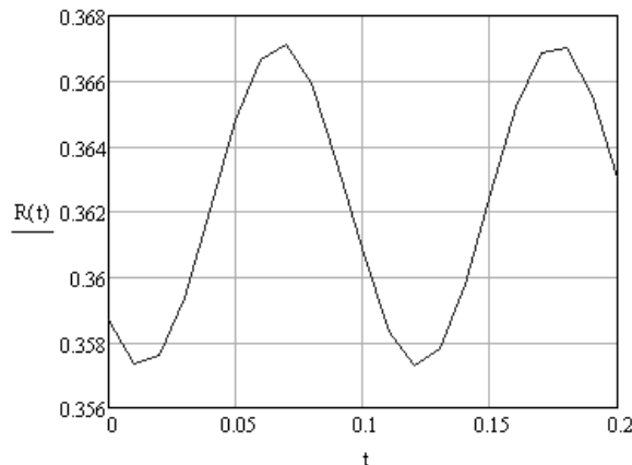
Рис. 5. Залежність радіуса шини від часу
