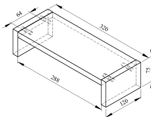
Рис. 1. Зразок кутового з'єднання корпуса на прохідних вертикальних стінках
